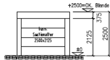
Vorderansicht
